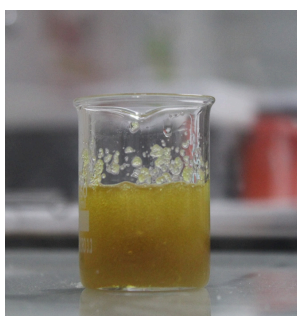
4- La réaction commence à libérer du gaz.
