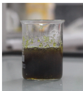
5- La tour de carbone commence à se former.
