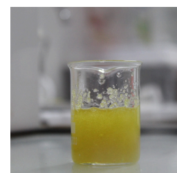
3- On mélange l'acide sulfurique avec le sucre. On peut apprécier que la réaction vient de débuter: le sucre devient jaunâtre et commence à disparaître.
